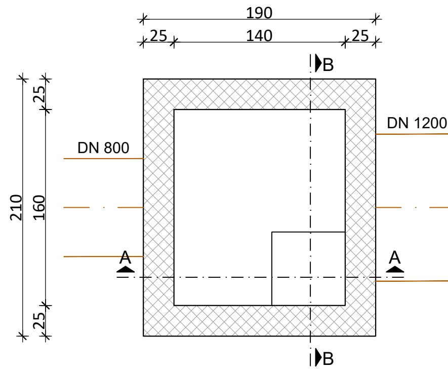
spoj DN 800 i DN 1200
